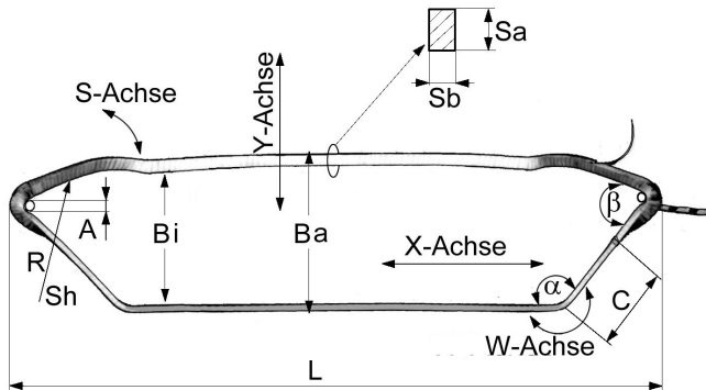
Abb.: Bandspule für Bandaufnahme / bobine à ruban pour prise du ruban
