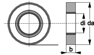
Abb.: Bandspule für Bandaufnahme / bobine à ruban pour prise du ruban
